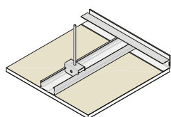
PERFIL PLADUR® T-45/T-60, HORQUILLAS, PIEZAS DE EMPALME Y CUELGUE
