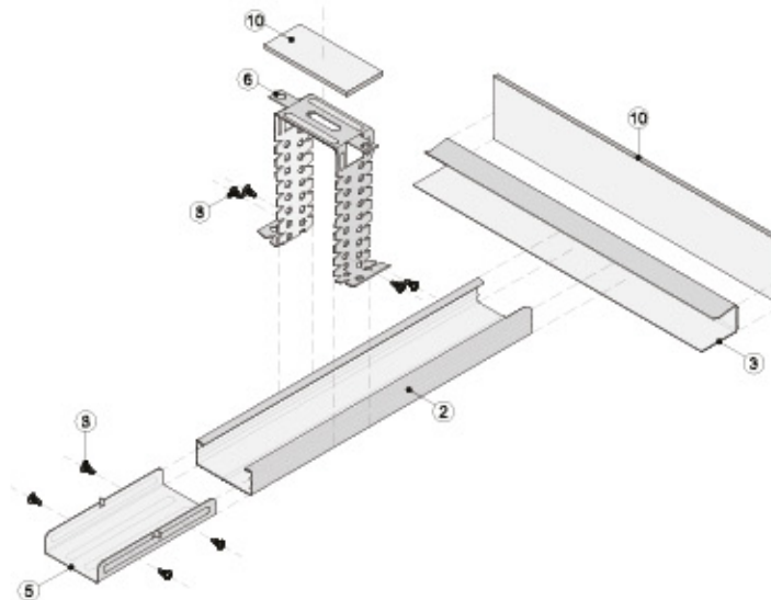
Vista isométrica
