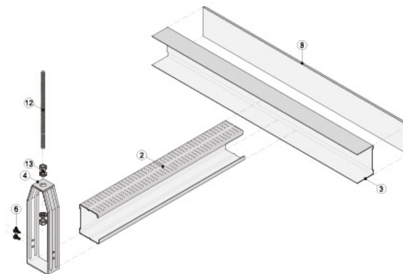
Vista isométrica
