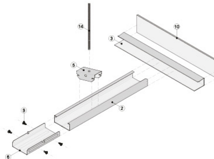
Vista isométrica
