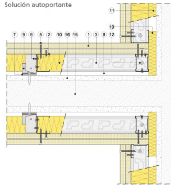
Sección horizontal
