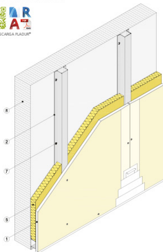
Vista isométrica
