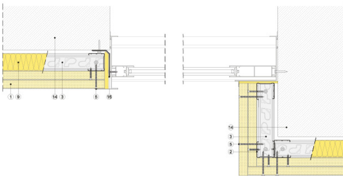
Sección horizontal
