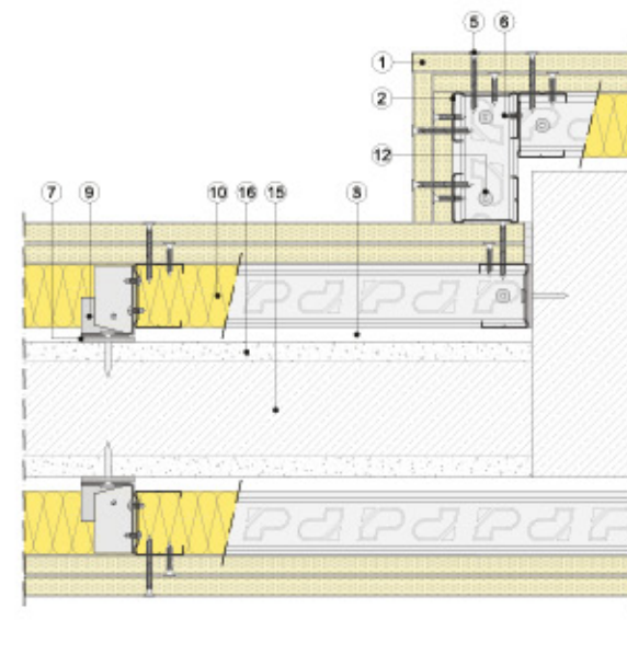
Sección horizontal
