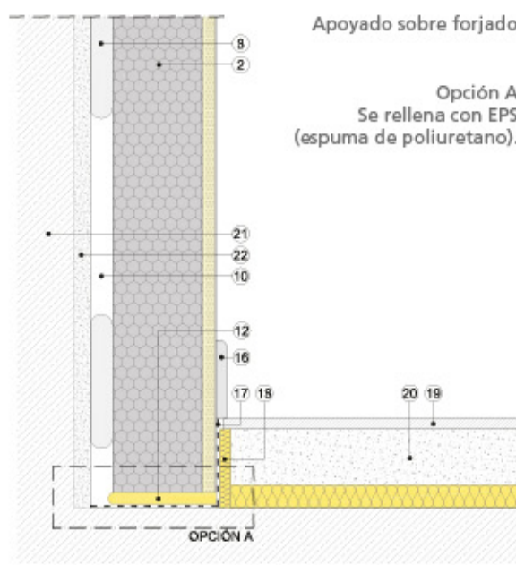
Sección vertical
