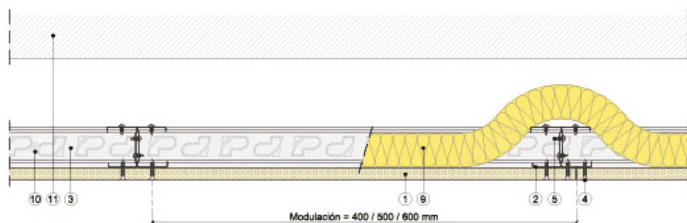
Sección vertical
