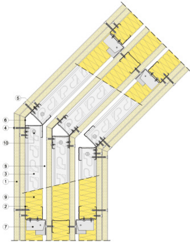
Sección horizontal
