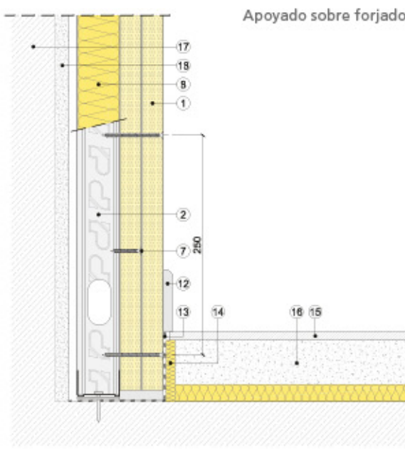
Sección vertical
