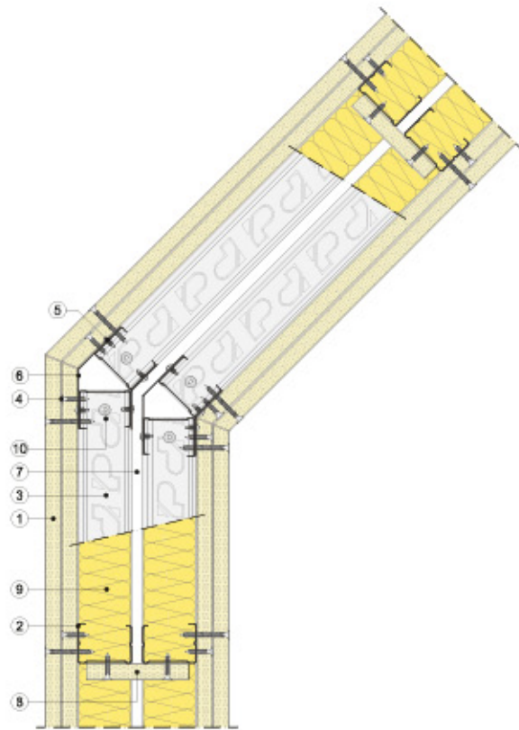
Sección horizontal
