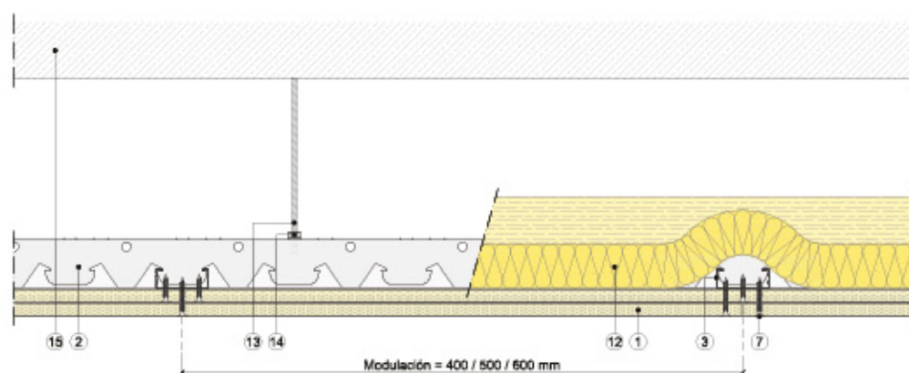
Sección vertical
