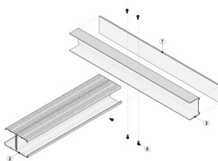
Vista isométrica
