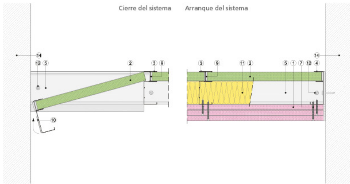
Sección horizontal
