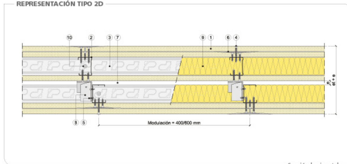
Sección horizontal
