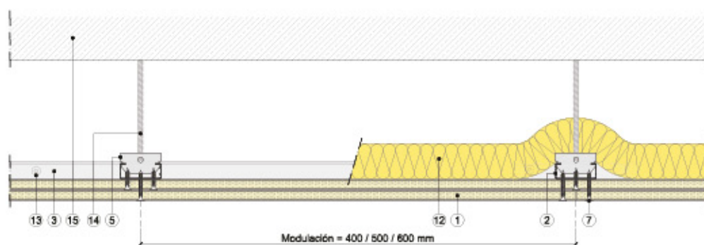
Sección vertical
