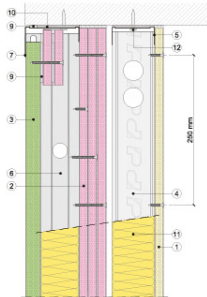
Sección vertical
