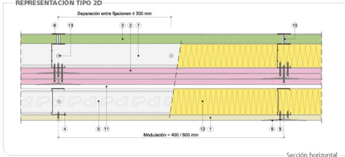
Sección horizontal
