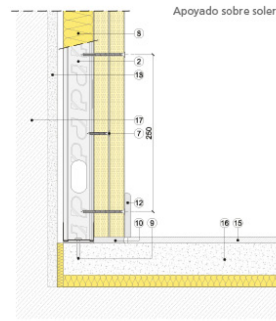
Sección vertical
