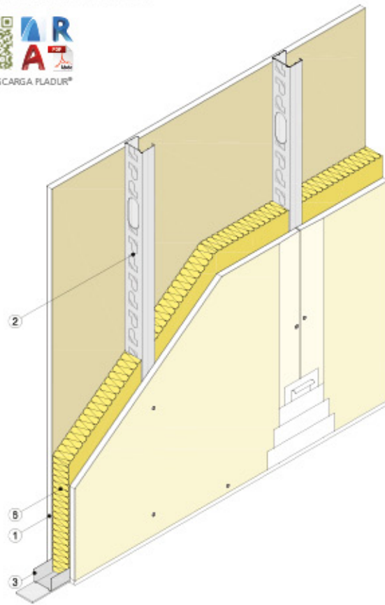
Vista isométrica
