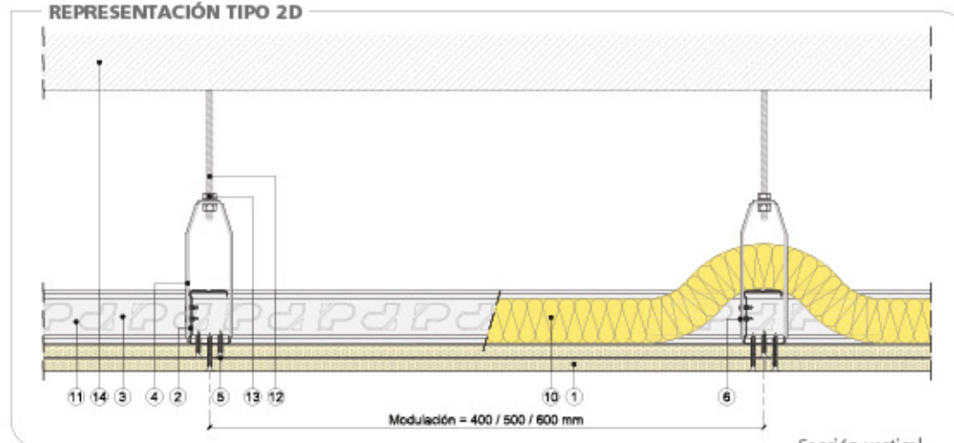
Sección vertical
