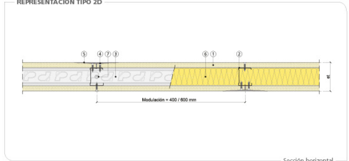
Sección horizontal
