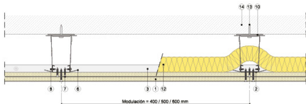
Sección vertical
