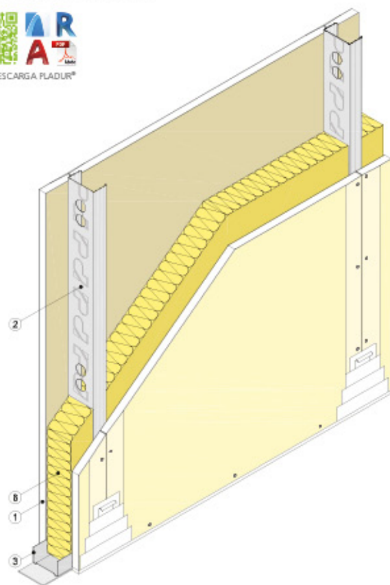
Vista isométrica
