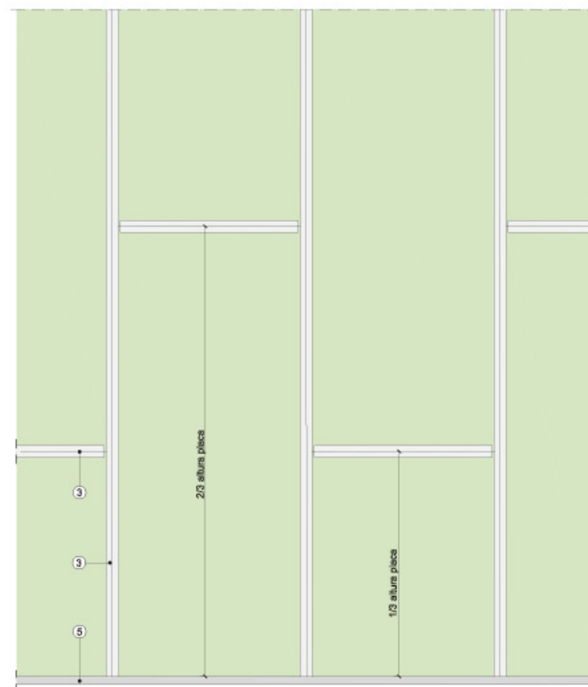
Sección vertical
