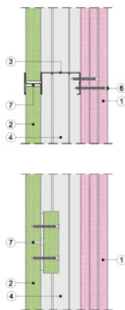
Sección vertical
