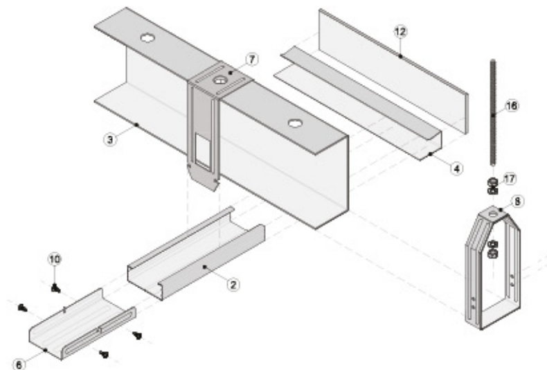
Vista isométrica
