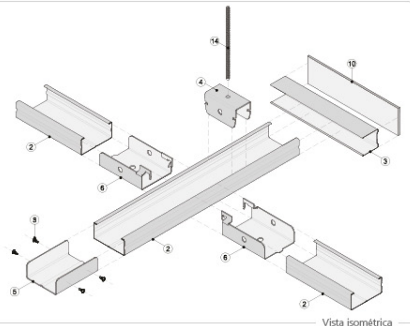
Vista isométrica
