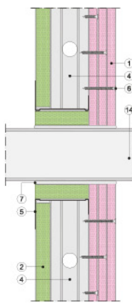
Sección vertical
