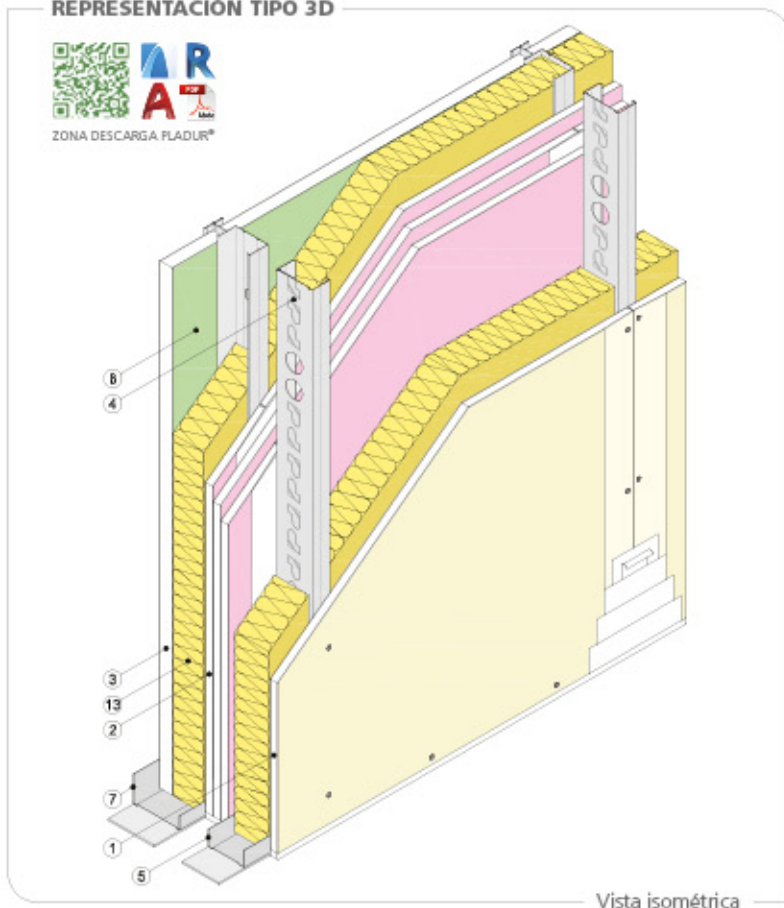
Vista isométrica
