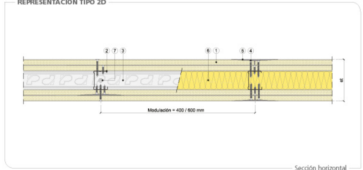
Sección horizontal
