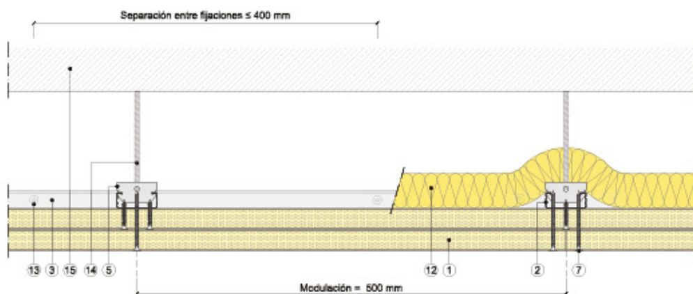
Sección vertical
