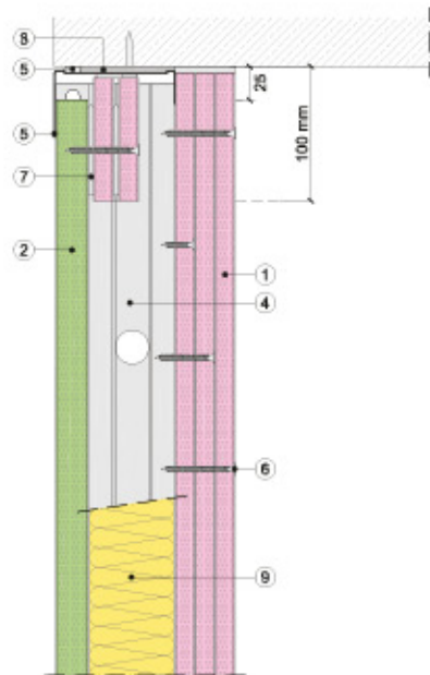
Sección vertical
