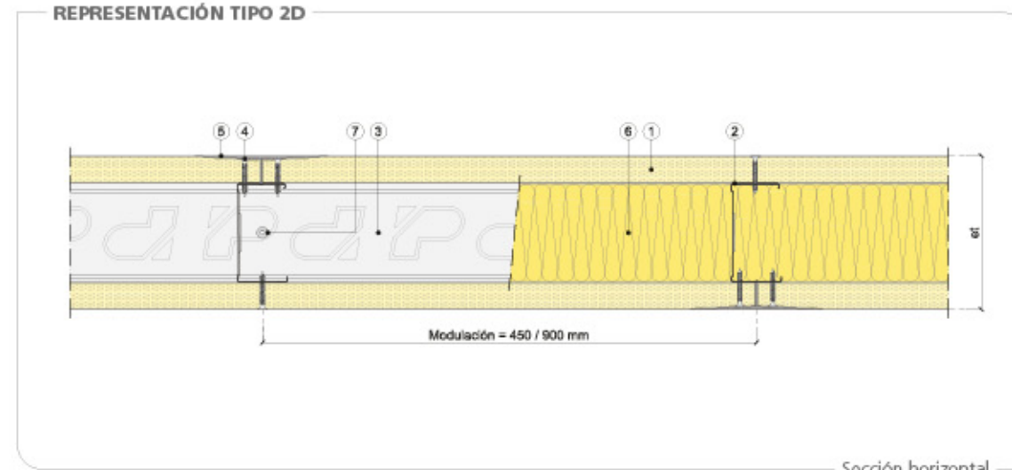
Sección horizontal
