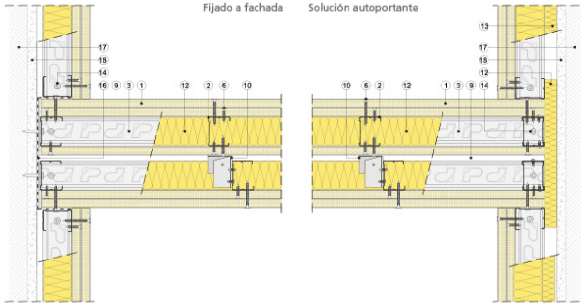
Sección horizontal
