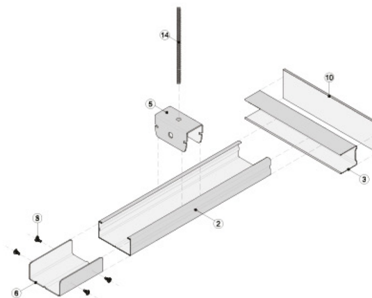
Vista isométrica
