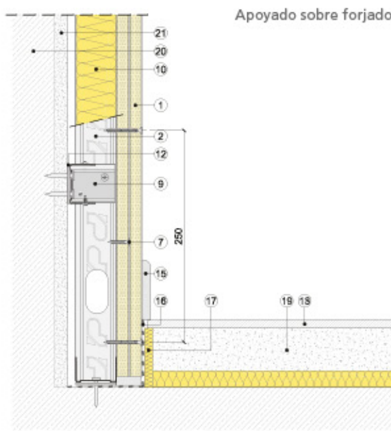
Sección vertical
