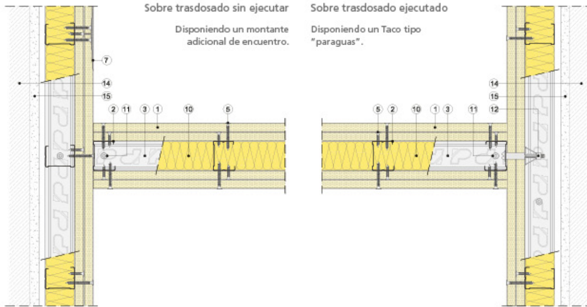
Sección horizontal
