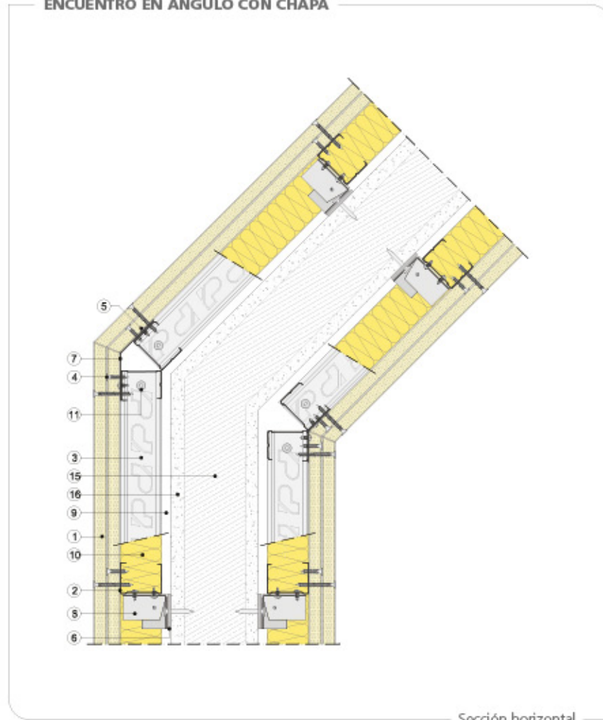
Sección horizontal
