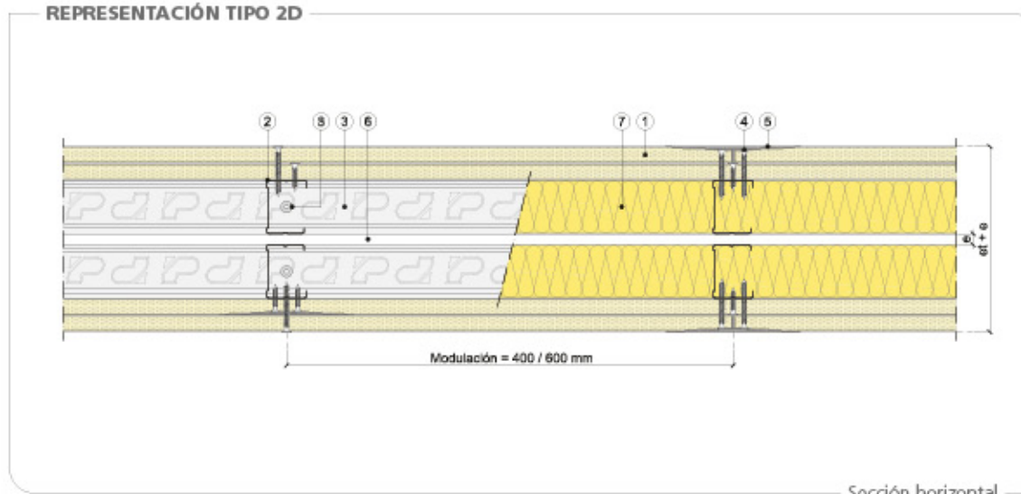
Sección horizontal
