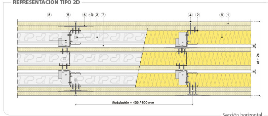
Sección horizontal
