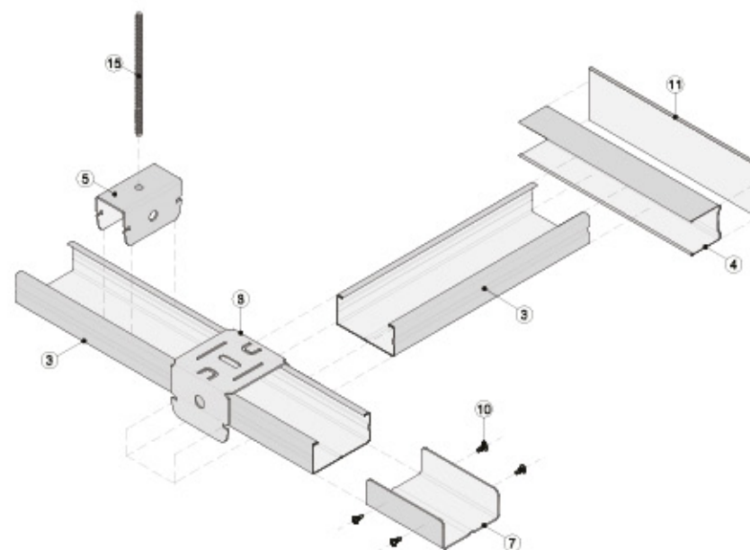
Vista isométrica
