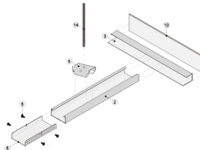
Vista isométrica
