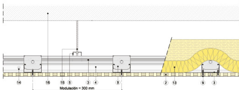
Sección vertical
