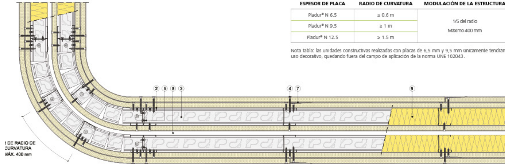
Sección horizontal
