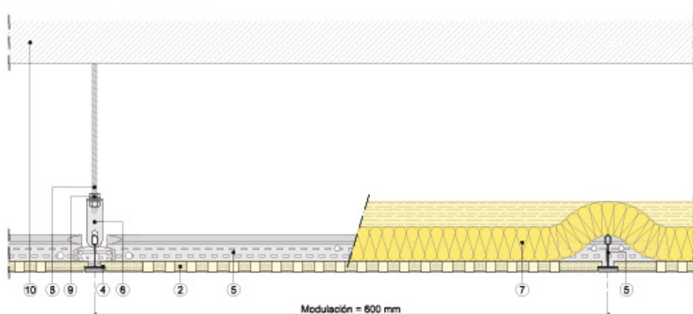
Sección vertical
