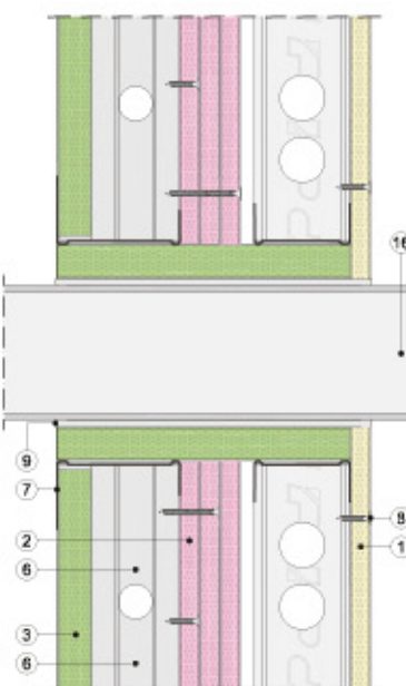
Sección vertical
