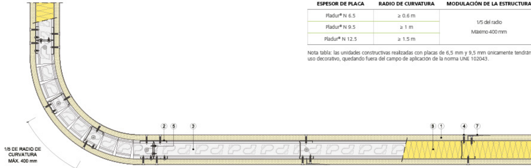
Sección horizontal
