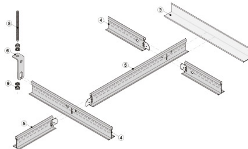
Vista isométrica
