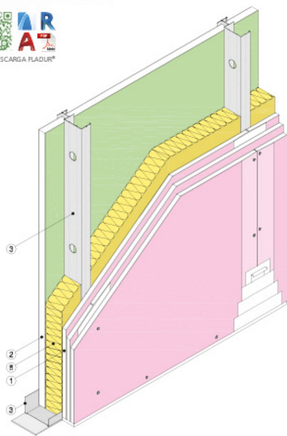
Vista isométrica
