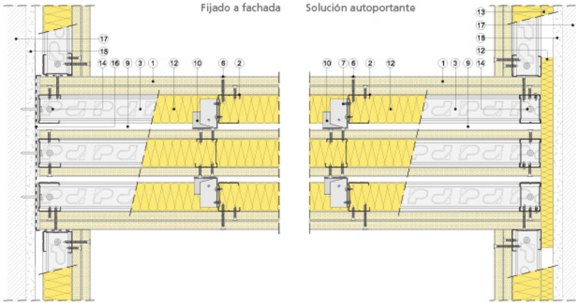
Sección horizontal
