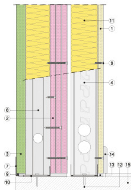
Sección vertical
