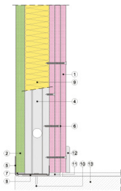
Sección vertical
