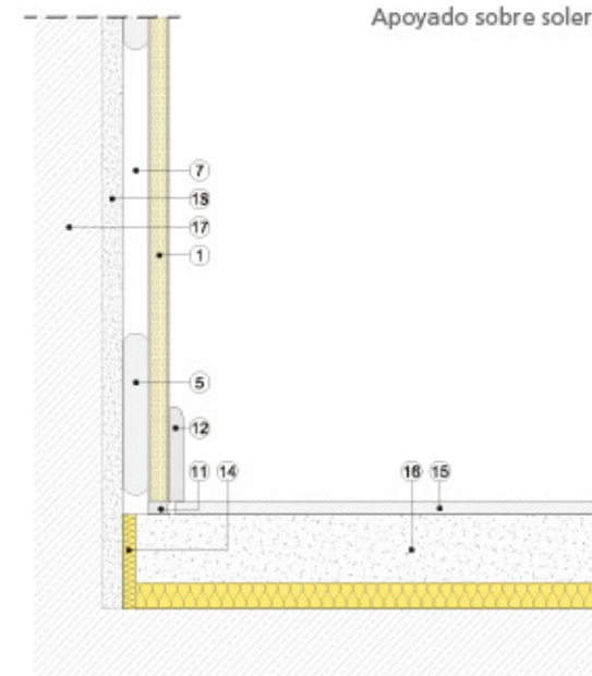
Sección vertical
