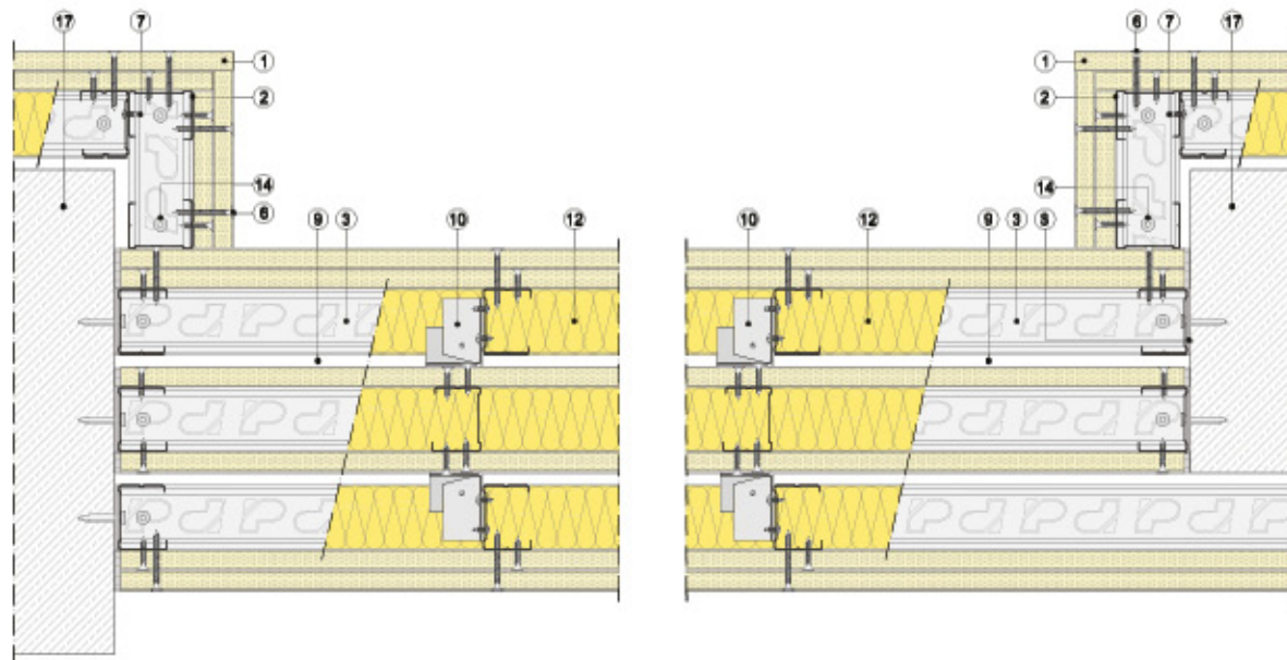
Sección horizontal
