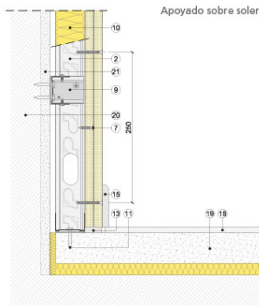
Sección vertical
