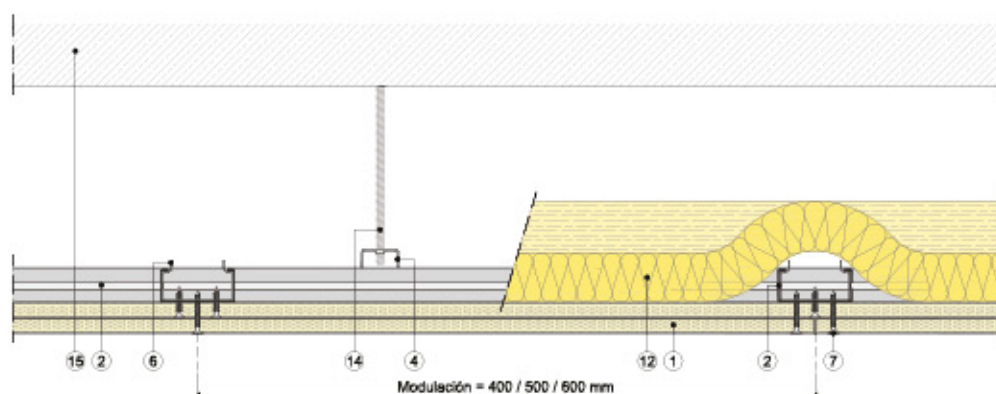
Sección vertical
