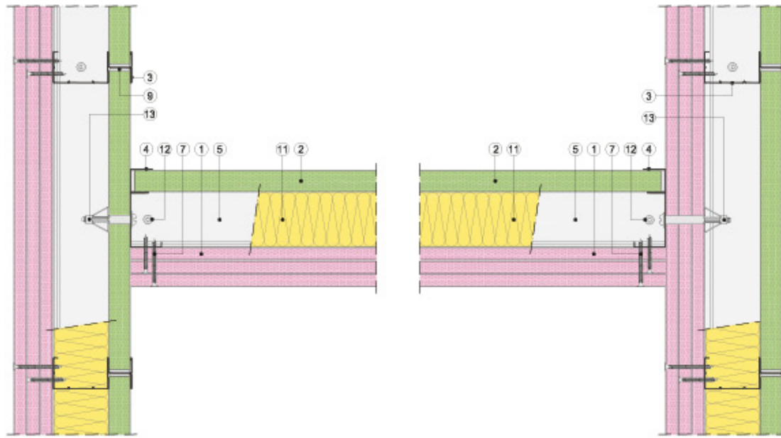
Sección horizontal
