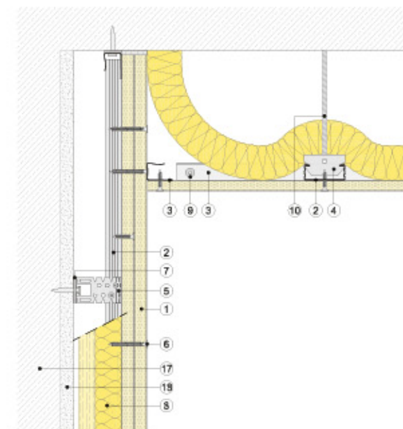
Sección vertical
