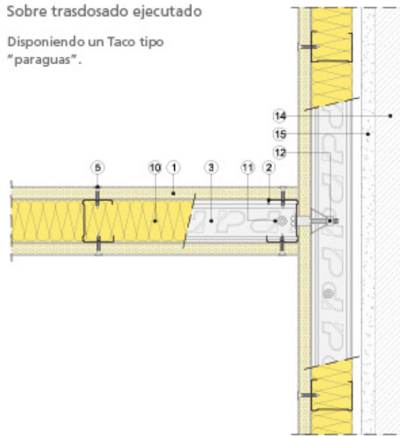
Sección horizontal
