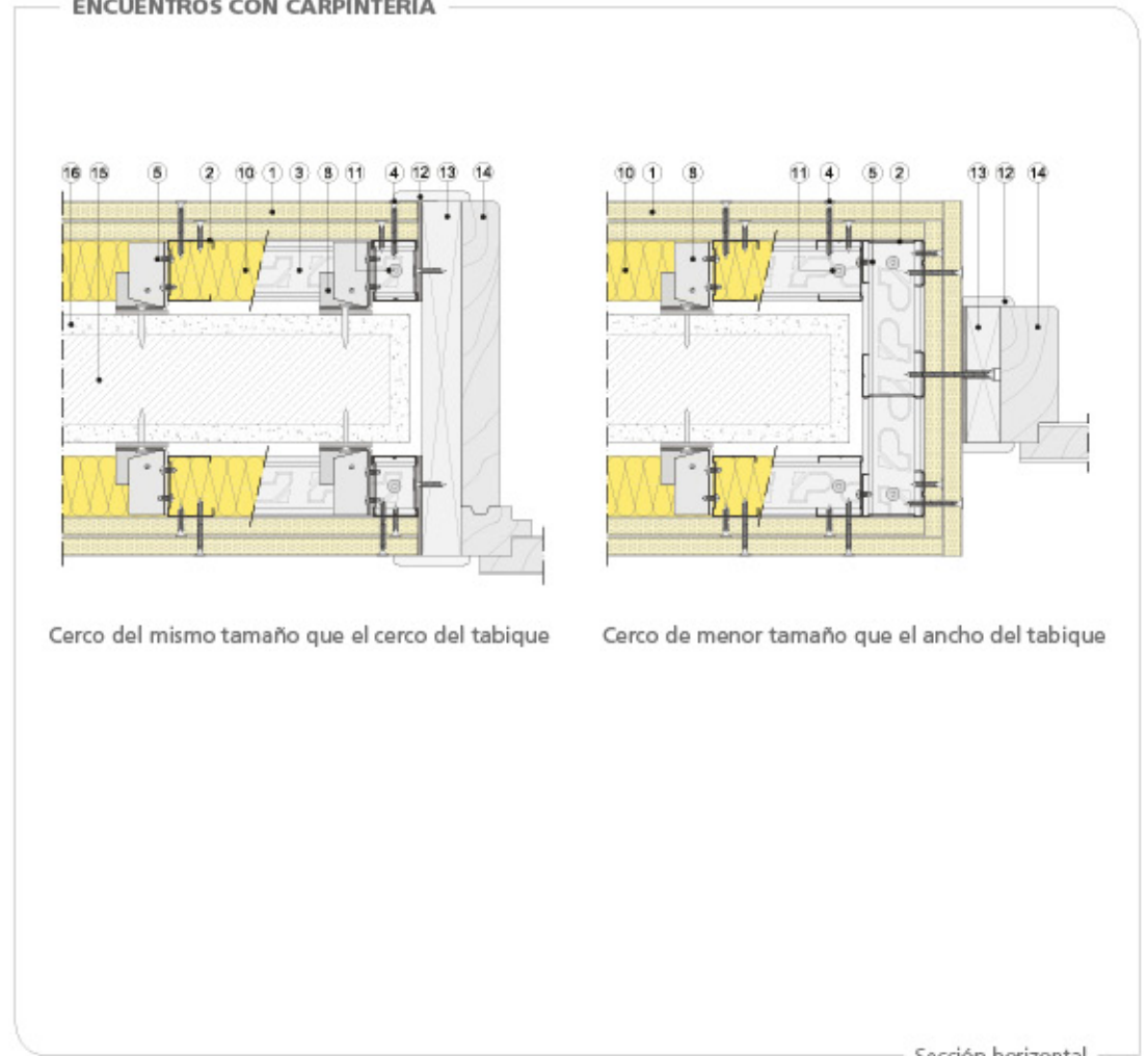
Sección horizontal
