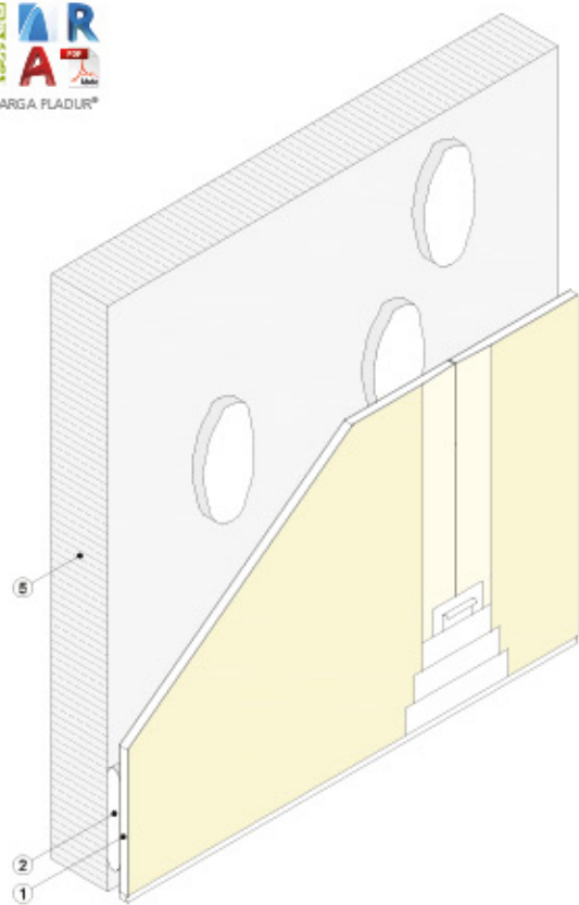
Vista isométrica
