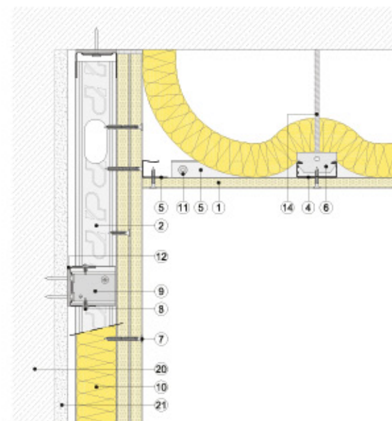
Sección vertical
