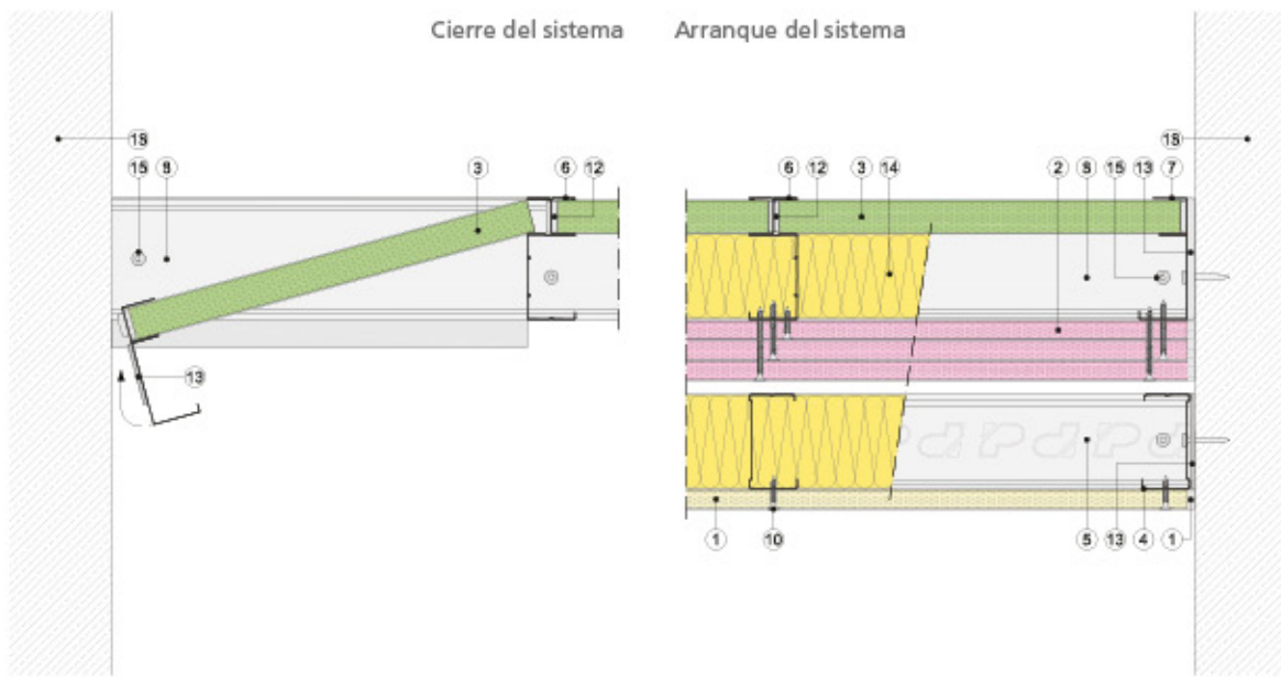
Sección horizontal
