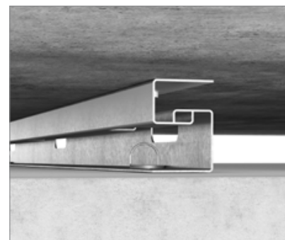
Es posible fijar la isla directamente al techo o forjado mediante el kit de suspensión directa para Rockfon Eclipse.
